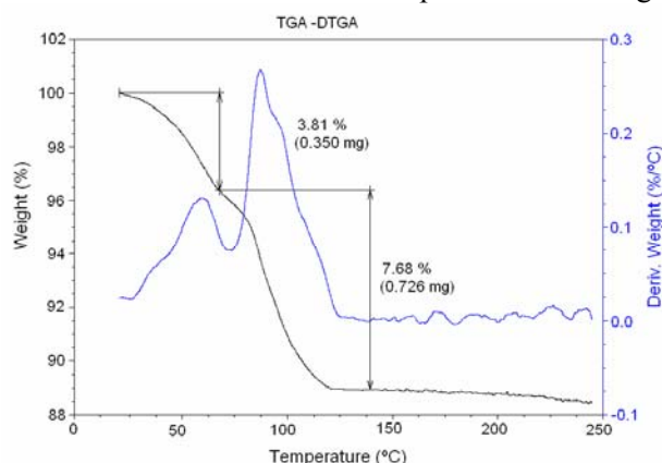
Figura 1. Curvas TGA-DTGA y DSC para el complejo K_3Fe(C_2O_4)_3 \cdot 3H_2O .
