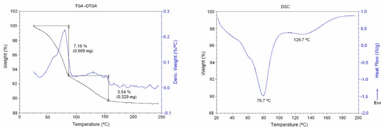
Figura 2. Curvas TGA-DTGA y DSC para el complejo K_3Cr(C_2O_4)_3 \cdot 3H_2O .
