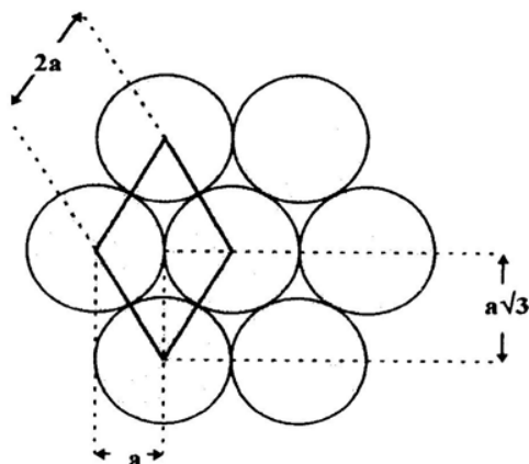
Figura 3. Representación de la estructura de empaquetamiento hexagonal de una monocapa de un tiol sobre una superficie de oro
