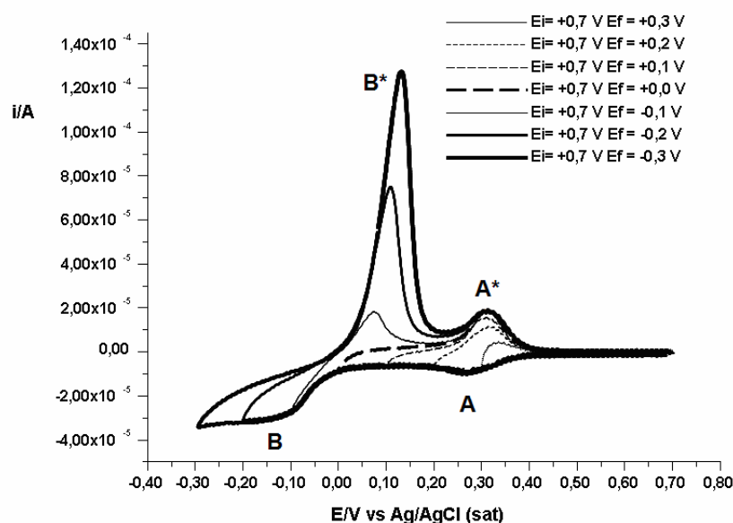
Figura 6. Familia de voltamperogramas cíclicos obtenidos en una solución reguladora acético/acetato (pH = 4,2) + 1 \times 10^{-2} M de iones Cu(II) con un electrodo de oro sin modificar
