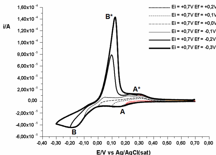
Figura 9. Familia de voltamperogramas cíclicos obtenidos en una solución reguladora acético/acetato (pH = 7,2) + 1 \times 10^{-2} M de iones Cu(II) con un electrodo de oro modificado con el ácido 2- N -bencil-1-ciclopenten-di-tiocarboxílico
