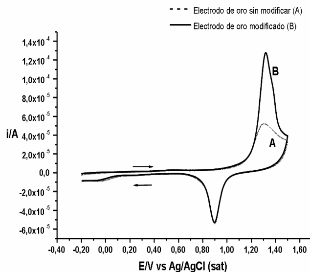
Figura 1. Voltamperogramas cíclicos obtenidos para: (A) electrodo de oro y (B) oro modificado químicamente en una solución de HClO_4 0,1 M. v = 200 \text{ mV s}^{-1} .
