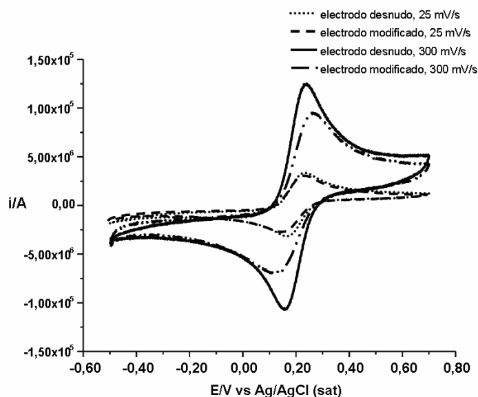
Figura 4. Familia de voltamperogramas cíclicos obtenidos en una solución reguladora acético/acetato ( \text{pH} = 4,2 ) + 1 \times 10^{-3} M de [\text{Fe}(\text{CN})_6]^{3-}/[\text{Fe}(\text{CN})_6]^{4-} con un electrodo de oro desnudo y modificado con el ácido 2- N -bencil-1-ciclopenten-di-tiocarboxílico a dos diferentes velocidades de barrido
