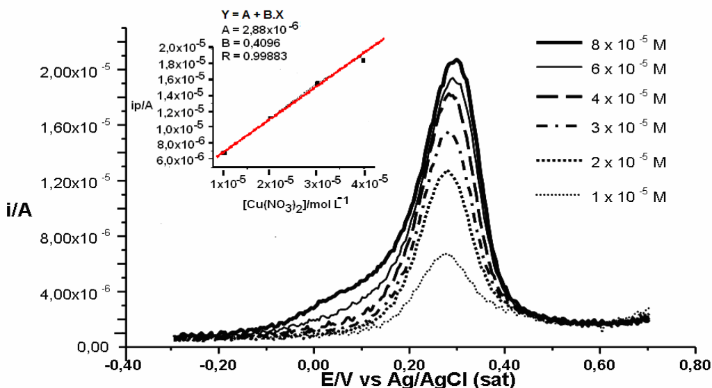
Figura 11. Familia de voltamperogramas obtenidos por VOCDA en una reguladora acético/acetato (pH = 7,2) con un electrodo de oro modificado después de su inmersión en solución reguladora acético/acetato (pH = 7,2) de concentración variable en iones Cu(II) y aplicación de un potencial de -0,25 V durante un tiempo determinado
