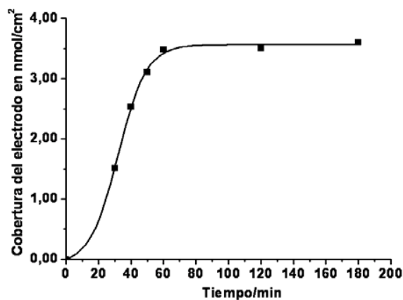
Figura 2. Comportamiento de la cobertura superficial del electrodo de oro en función del tiempo que se sumerge en una solución saturada de ácido 2- N -bencil-1-ciclopenten-di-tiocarboxílico en cloroformo
