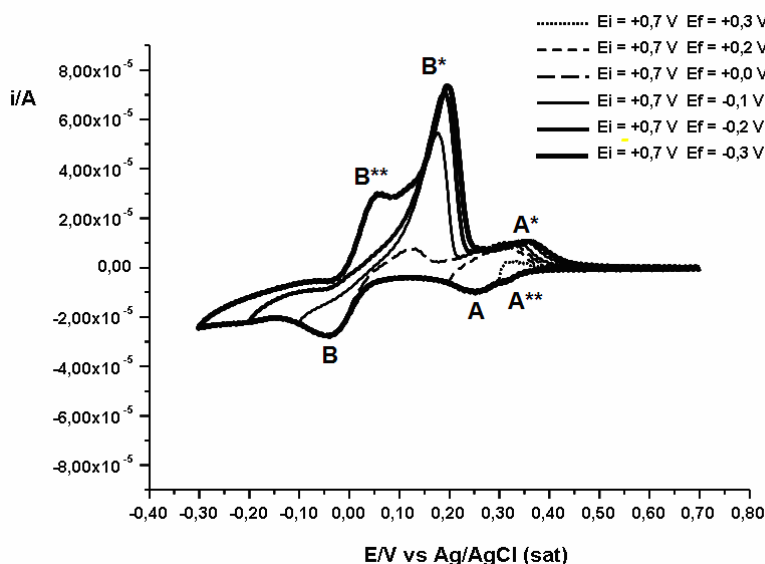
Figura 8. Familia de voltamperogramas cíclicos obtenidos en una solución reguladora acético/acetato (pH 7,2) + 1 \times 10^{-2} M de iones Cu(II) con un electrodo de oro sin modificar
