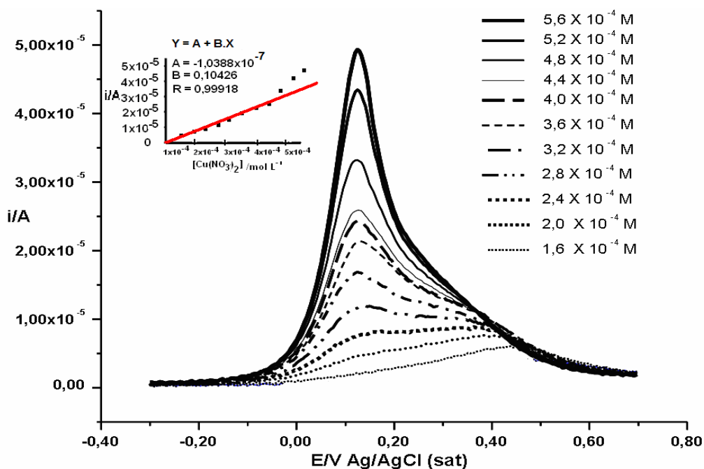
Figura 9. Familia de voltamperogramas cíclicos obtenidos en una solución reguladora acético/acetato (pH = 7,2) + 1 \times 10^{-2} M de iones Cu(II) con un electrodo de oro modificado con el ácido 2- N -bencil-1-ciclopenten-di-tiocarboxílico
