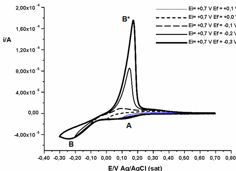
Figura 7. Familia de voltamperogramas cíclicos obtenidos en una solución reguladora acético/acetato (pH = 4,2) + 1 \times 10^{-2} M de iones Cu(II) con un electrodo de oro modificado con el ácido 2-N-bencil-1-ciclopenten-di-tiocarboxílico
