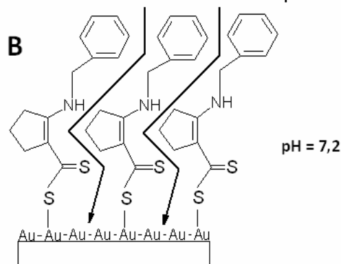
Esquema 1. Comportamiento de la monocapa autoensamblada del ácido 2-N-bencil-1-ciclopenten-di-tiocarboxílico a \text{pH} ácido y \text{pH} básico.
