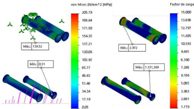
Fig. 12. Resultados de tensión de von Mises para Fcmáx y del Factor de Carga en el estudio de fatiga para el acero en la condición II.
