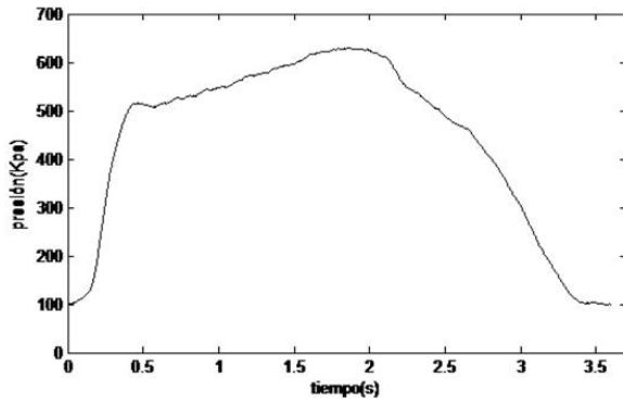
Fig. 13. Curva P-t prueba número tres.
