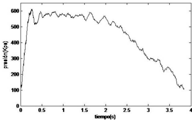
Fig. 9 Curva P-t prueba número dos.
