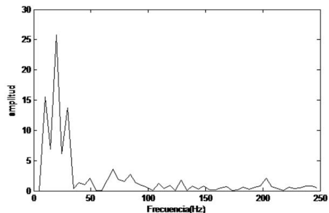
Fig. 7. PSD entre 0,8 y 1 s, prueba número uno.
