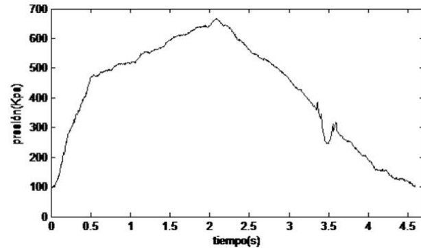
Fig. 5. Curva P-t prueba número uno.
