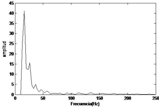
Fig. 8. PSD entre 3,35 y 3,65 s, prueba número uno.
