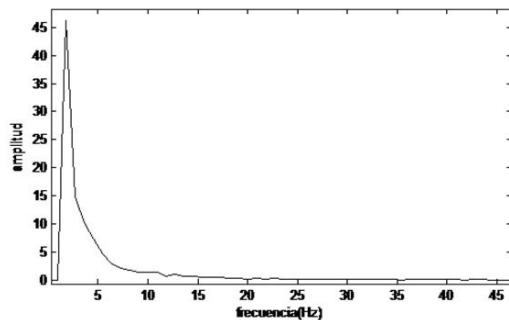
Fig. 15. PSD entre 0,75 y 1,85 s prueba número tres.
