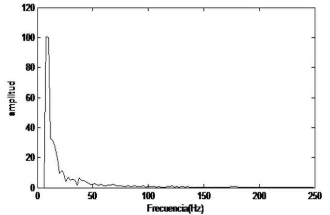
Fig. 11. PSD entre 0 y 0,5 s prueba número dos.
