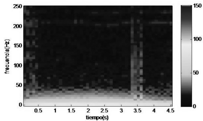
Fig. 6. Espectrograma curva P-t prueba número uno.
