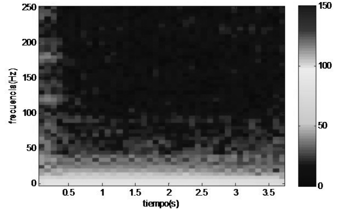
Fig. 10. Espectrograma curva presión versus tiempo, prueba número dos.
