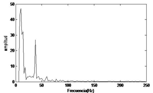
Fig. 12. PSD entre 1 y 1,5 s prueba número dos
