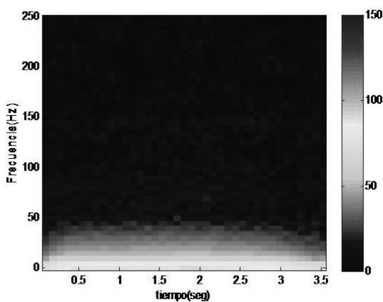
Fig. 14. Espectrograma curva presión versus tiempo, prueba número tres.
