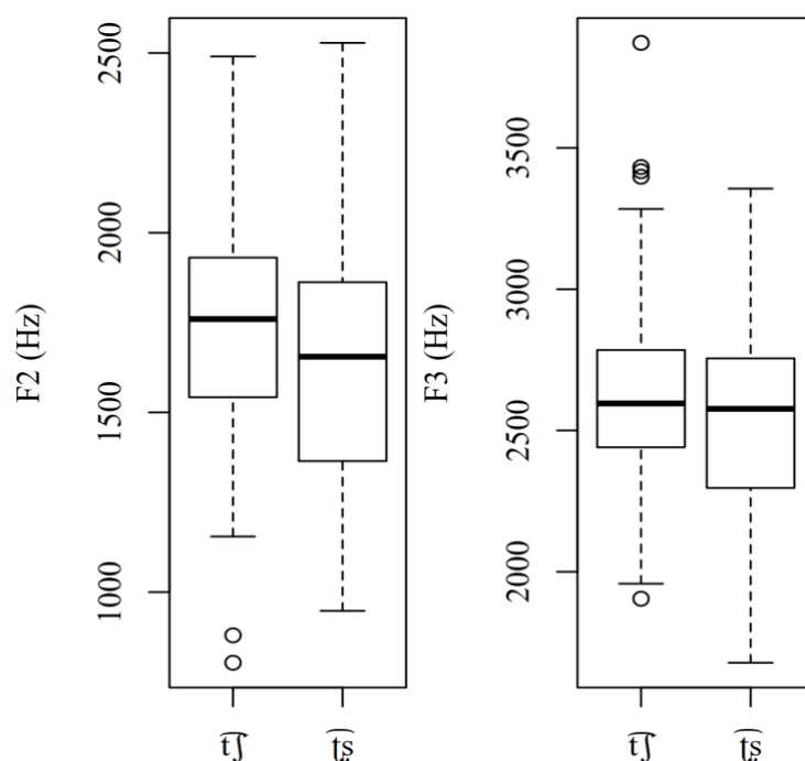
Figura 2. Panel izquierdo: gráficos de caja para los valores de F2 previos en las consonantes \widehat{tj} y \widehat{t\ddot{s}} . Panel derecho: gráficos de caja para los valores de F3 previos en las consonantes \widehat{tj} y \widehat{t\ddot{s}} .
