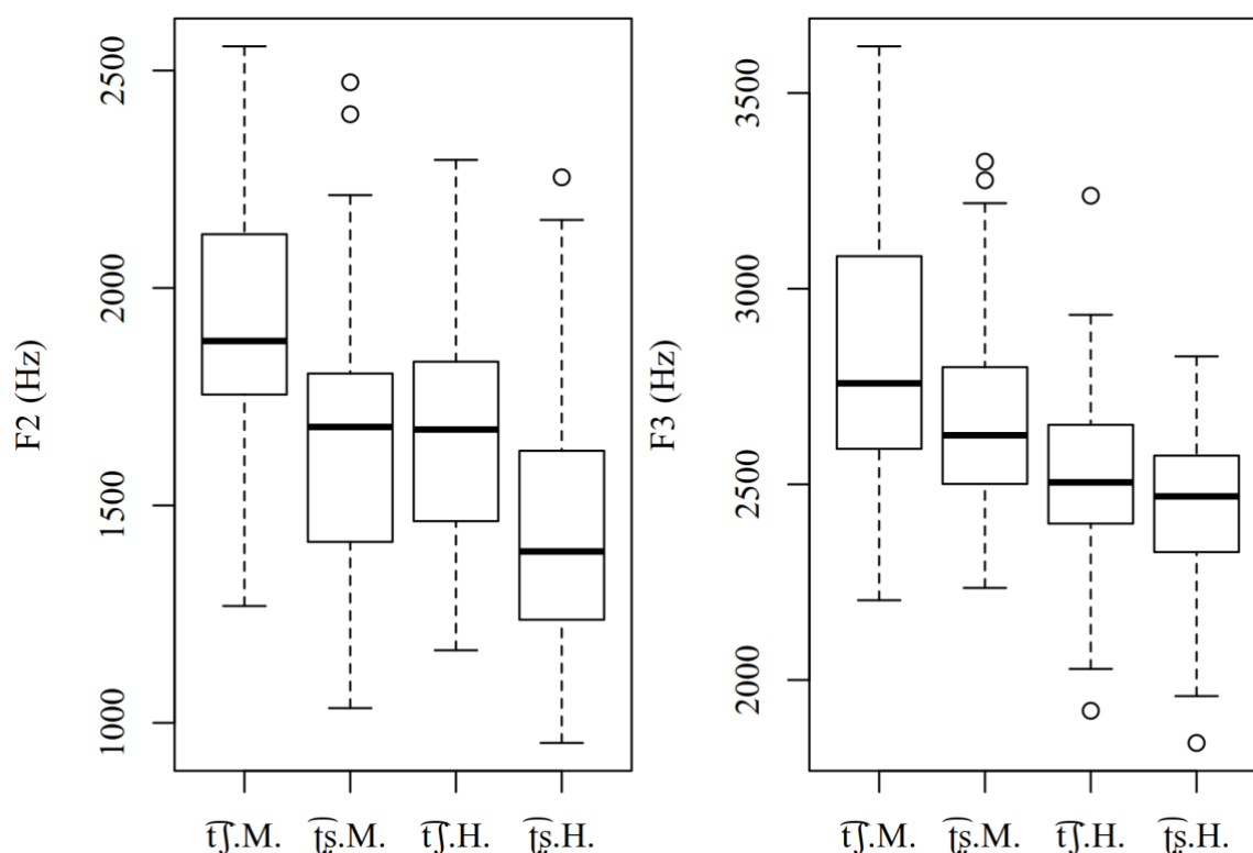
Figura 11. Panel izquierdo: gráfico de cajas con las distribuciones de F2 siguientes para las consonantes /tʃ/ y /tʂ/ separadas por sexo (“M” = mujer, “H” = hombre). Panel derecho: gráfico de cajas con las distribuciones de F3 siguientes para las consonantes /tʃ/ y /tʂ/ separadas por sexo (“M” = mujer, “H” = hombre).
