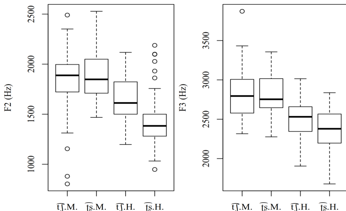
Figura 6. Panel izquierdo: gráfico de cajas con las distribuciones de F2 previas para las consonantes /tʃ/ y /tʂ/ separadas por sexo (“M” = mujer, “H” = hombre). Panel derecho: gráfico de cajas con las distribuciones de F3 previas para las consonantes /tʃ/ y /tʂ/ separadas por sexo (“M” = mujer, “H” = hombre).
