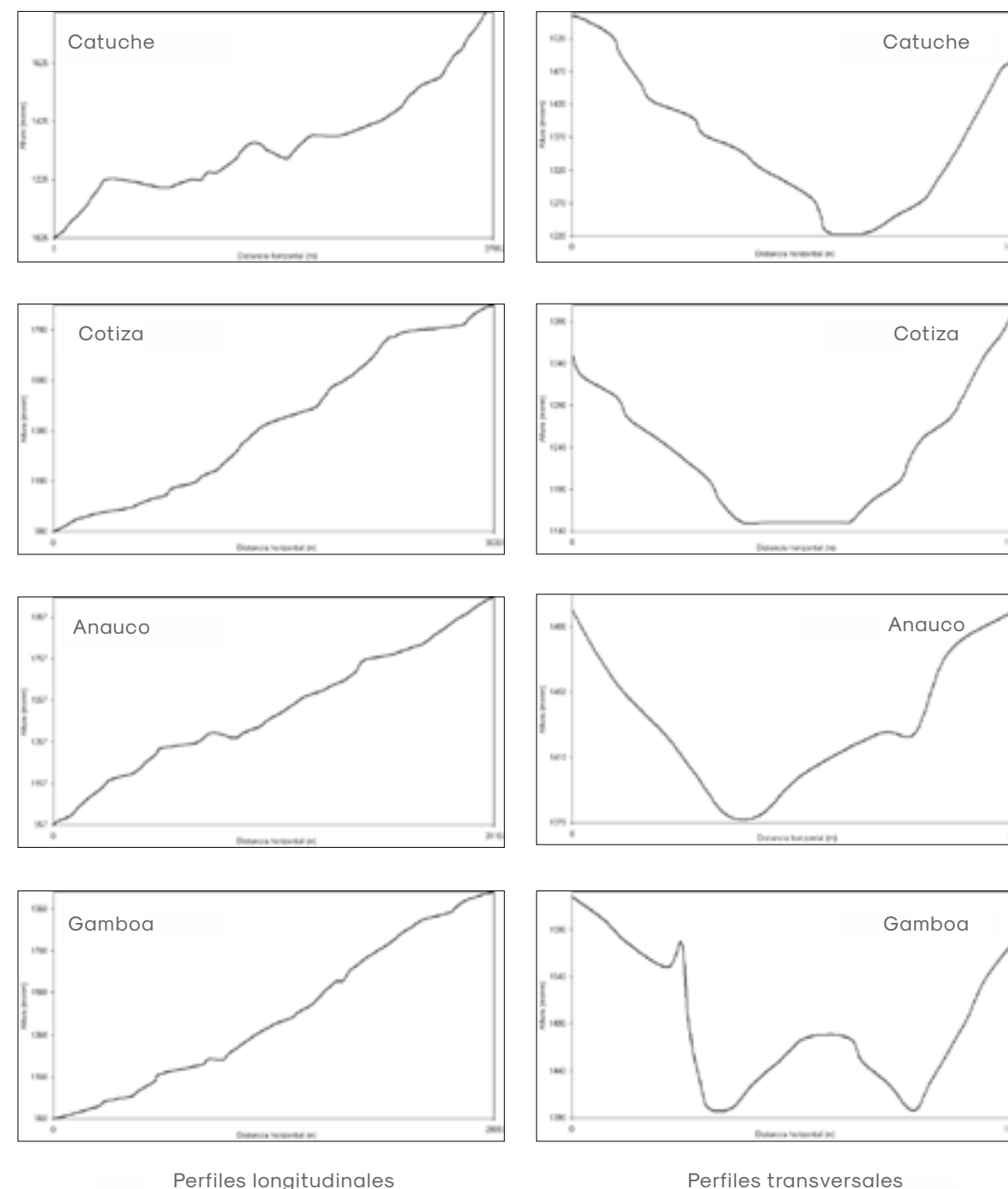
Figura 4. Perfiles topográficos longitudinales y transversales (cuencas medias) de las microcuencas de drenaje
