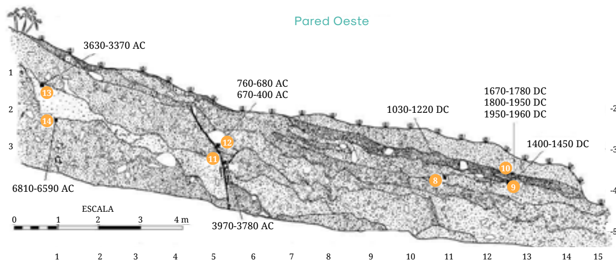
Figura 8. Estratigrafía de la pared oeste de la trinchera Santa Rosa, con la ubicación de los sitios de muestras datadas por C 14 , para facilitar su comparación con la pared este, esta pared es imagen especular de la original.
