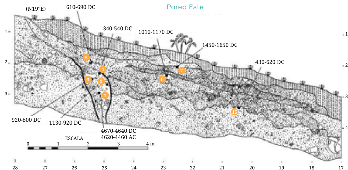
Figura 7. Estratigrafía de la pared este de la trinchera Santa Rosa y ubicación de los sitios de muestras datadas por C 14 .
