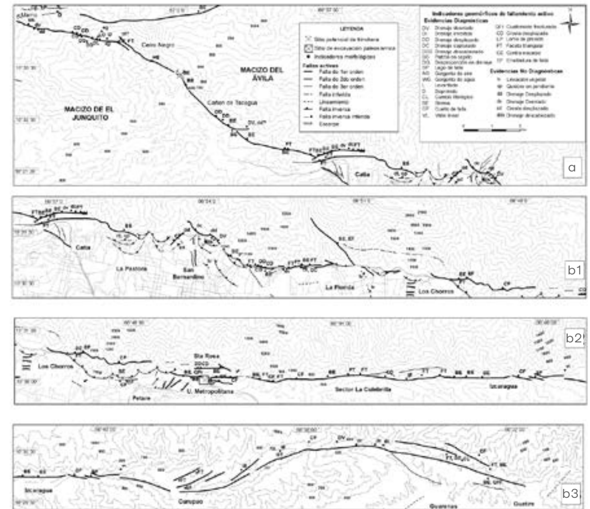
Figura 2. Trazado del sistema de fallas Tacagua-El Ávila. Evidencias morfológicas de actividad tectónica reciente. (a) segmento Tacagua, desde la cercanía de Mamo hasta Catia; (b1) segmento Ávila, sección entre Catia y Los Chorros, (b2) segmento Ávila, sección entre Los Chorros hasta Izcaragua, (b3) segmento Ávila, sección entre Izcaragua y Guatire.
