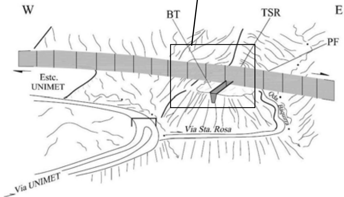
Figura 5. Ubicación del sitio de excavación paleosísmico en Santa Rosa. BT: berma tectónica, PF: plano de falla, TSR: trinchera paleosísmica, UNIMET: Estacionamiento Universidad Metropolitana. Foto: Audemard, 2007
